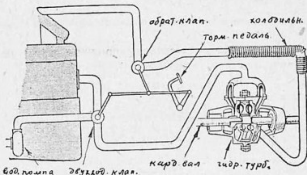
Рис. 2. Система Кюрна для регулировки температуры в двигателе
